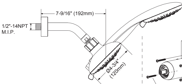
Shower arm / Bras de douche Shower head / Pomme de douche
